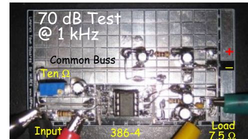
9 V, 1.275 uVpp input, Output ~350 mW @12 V, ~800 mW
